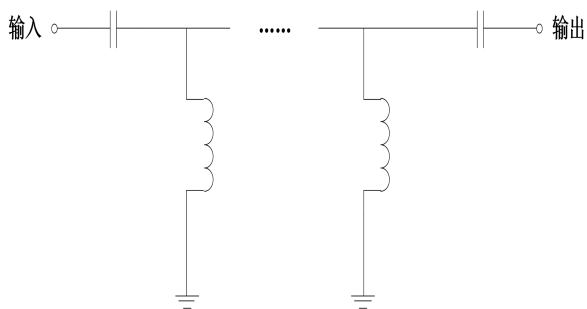
YLLP-1400-D4-W7.8产品原理图
